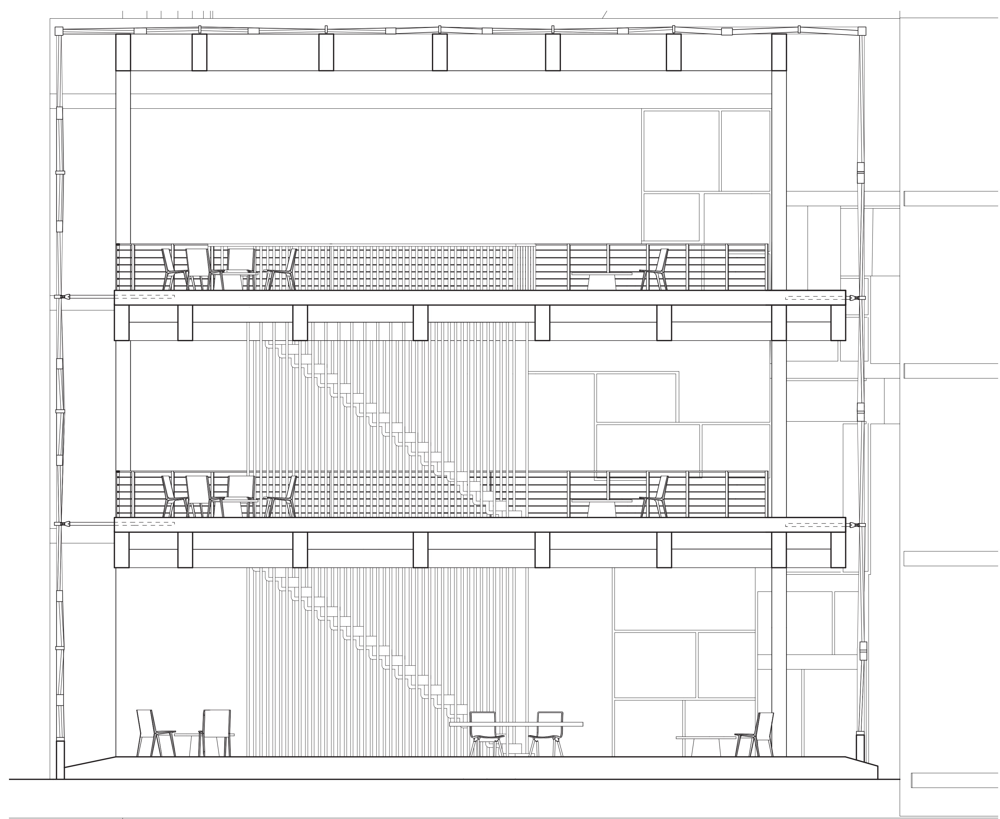
SECTION | SCALE: 1/4" = 1'-0"
