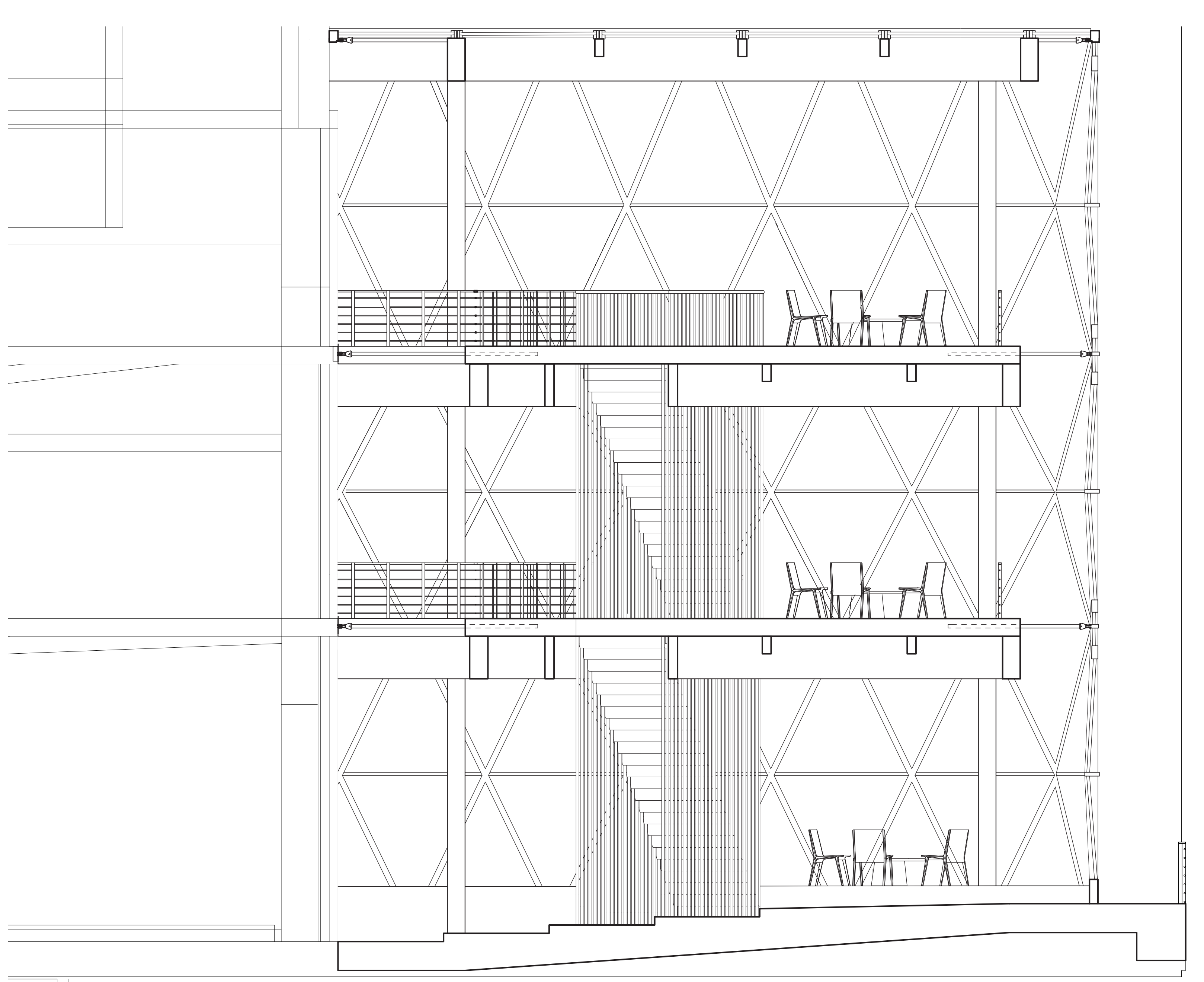
SECTION | SCALE: 1/4" = 1'-0"
